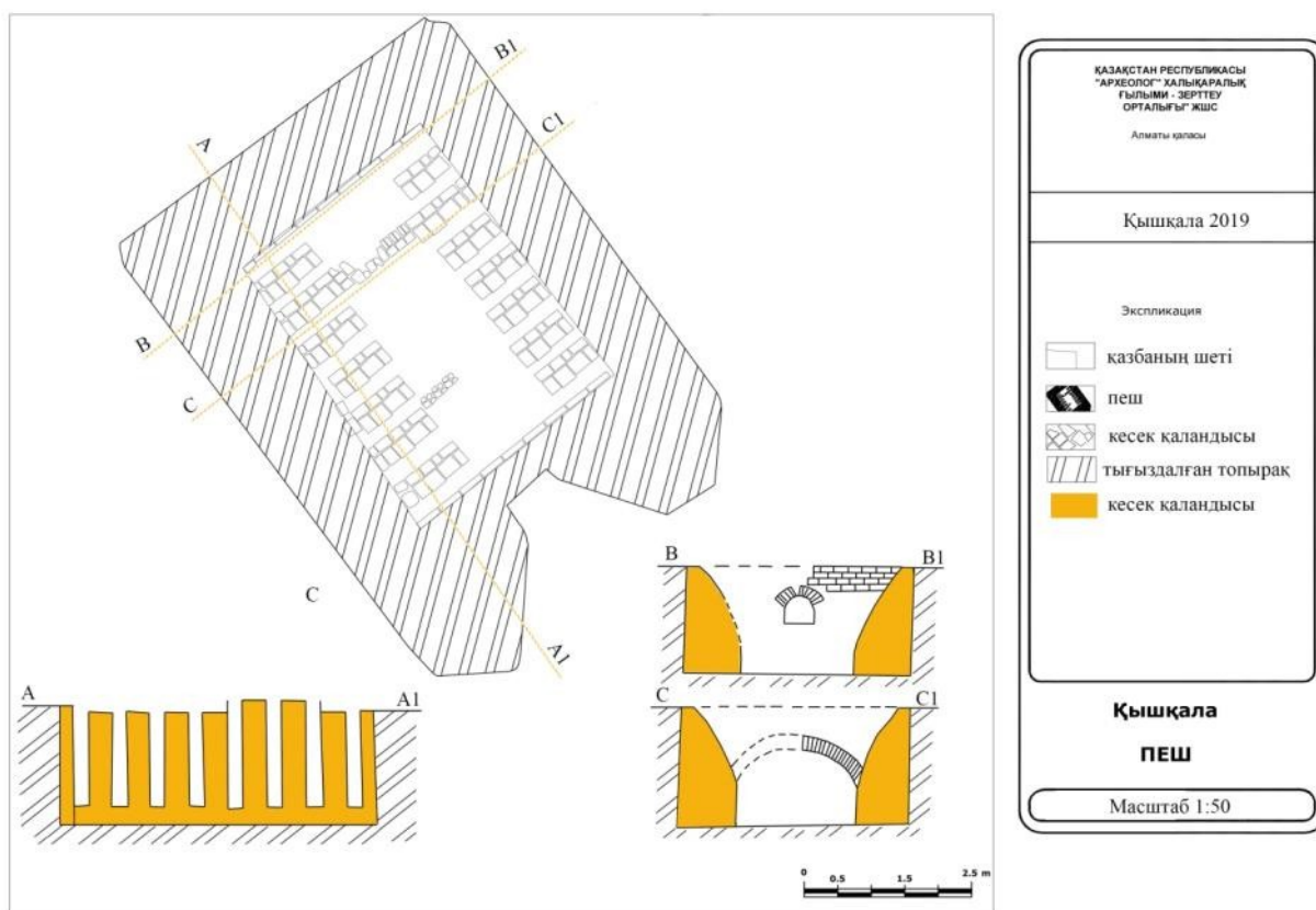
Сурет А.33 – Қыш күйдіретін пештің жобасы мен кесіндісі
